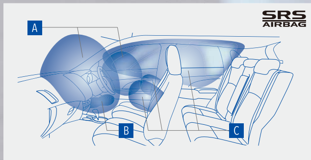
各エアバッグ展開イメージ
