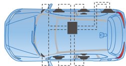
スピーカー・ハイパワーアンプ配置図
