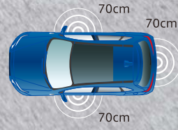
ドアエントリーの有効エリア
